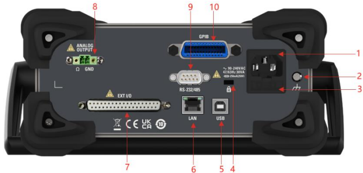
图 4.5 后面板
