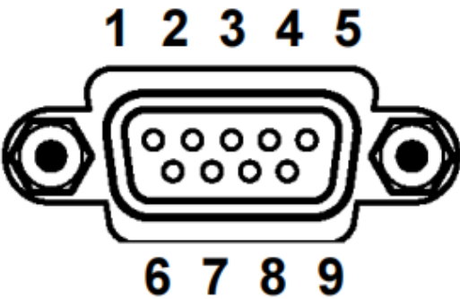
图 9.5 RS232/485 连接器
